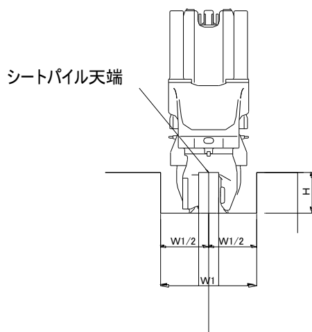
布 掘 寸 法 表
