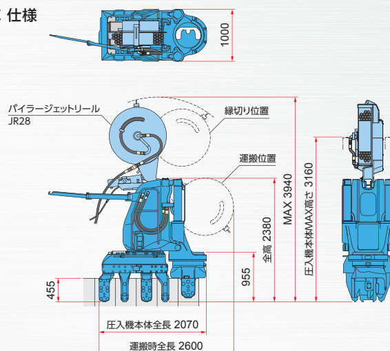
圧入機本体
