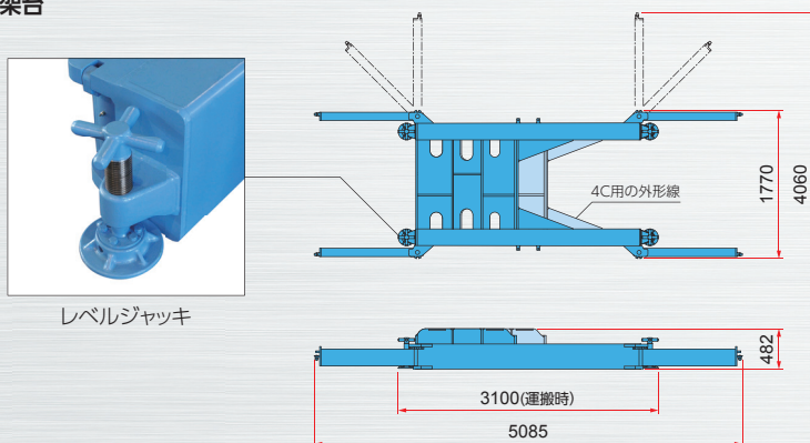
反力架台
